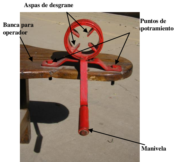
Desgranadora de maíz manual, listo para iniciar su trabajo
