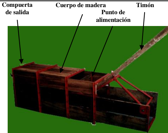
Enfardadora de madera, listo para iniciar su trabajo de elaboración de heno
