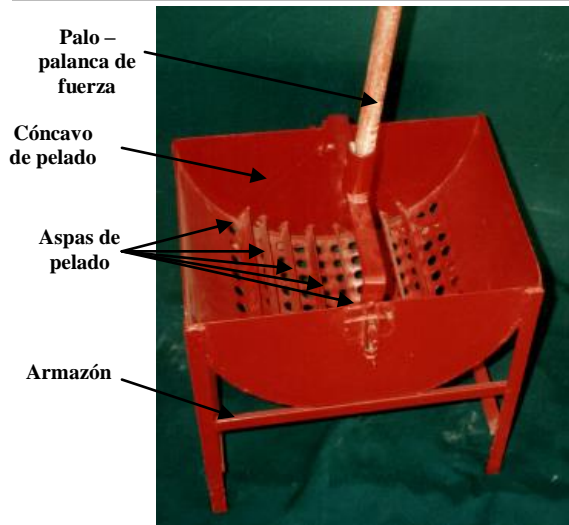
Peladora de maní, listo para iniciar su trabajo de pelado o desvainado
