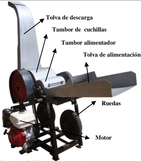
Picadora P-80 sin tapa, se observa sus partes principales
