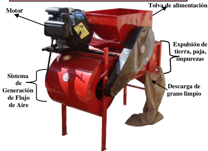
Venteadora V-1, limpia varios tipos de granos sean de cereales como de leguminosas u otros
